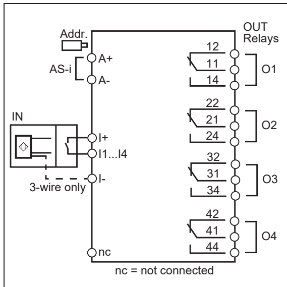
Fig. 5: Wiring
