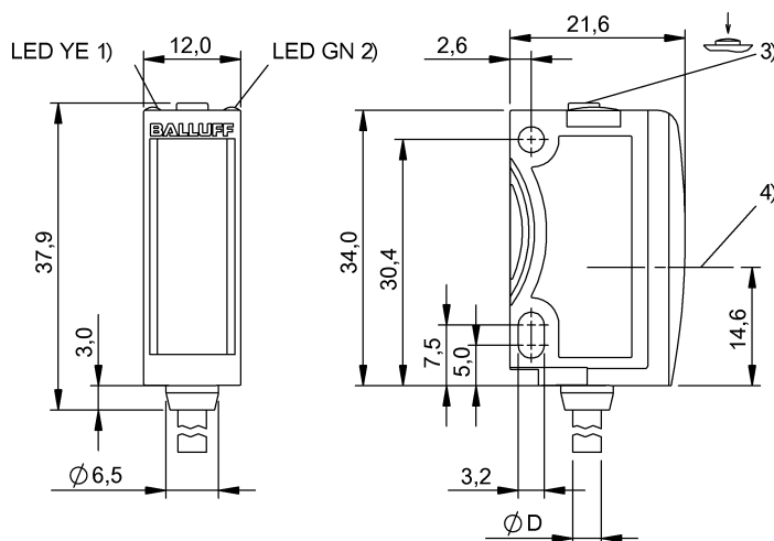
1) Funkcja wyjścia 2) Napięcie robocze 3) Czulość, jasno/ciemno 4) Oś optyczna
