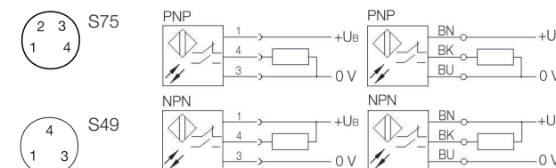
Bild 3: Anschluss-Schaltbild, Steckerbild
