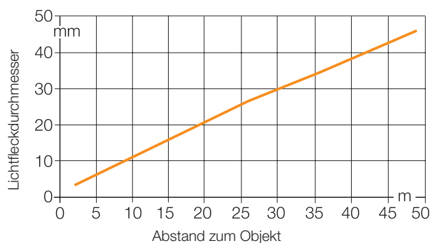
Bild 5: Lichtfleckdurchmesser in Abhängigkeit vom Objekt-abstand
