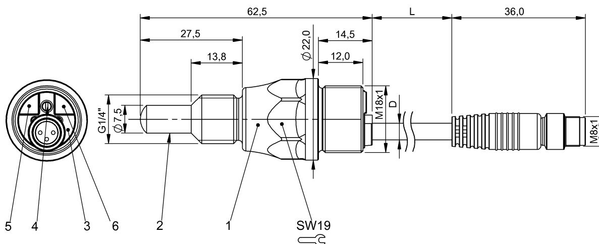
1) Obudowa 2) powierzchnia aktywna 3) Pokrywa 4) Potencjometr 5) Wskazanie funkcji żółty 6) Wskaźnik napięcia roboczego, zielony
