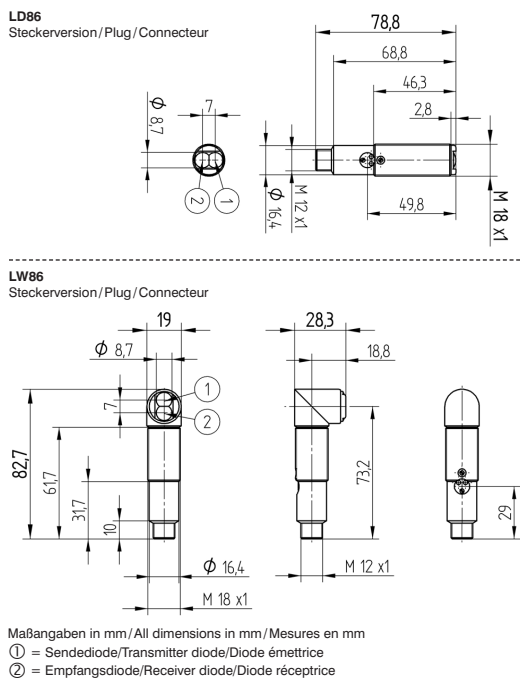
Spiegelreflexschranke Retro-Reflex Sensor Barrage sur réflecteur
