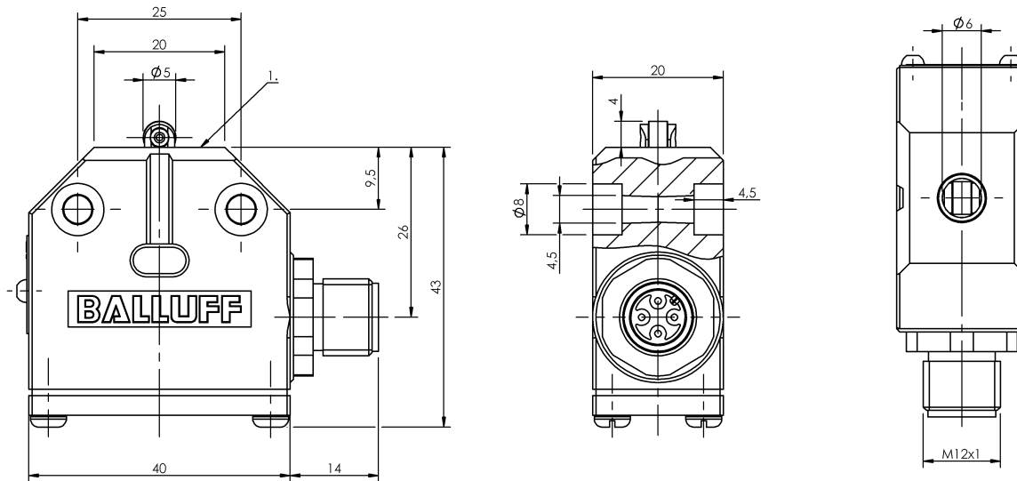
1) Krawędź odniesienia
