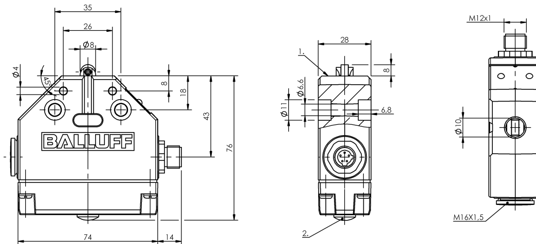
1) Krawędź odniesienia 2) Wskazanie funkcji FD/FE/LL
