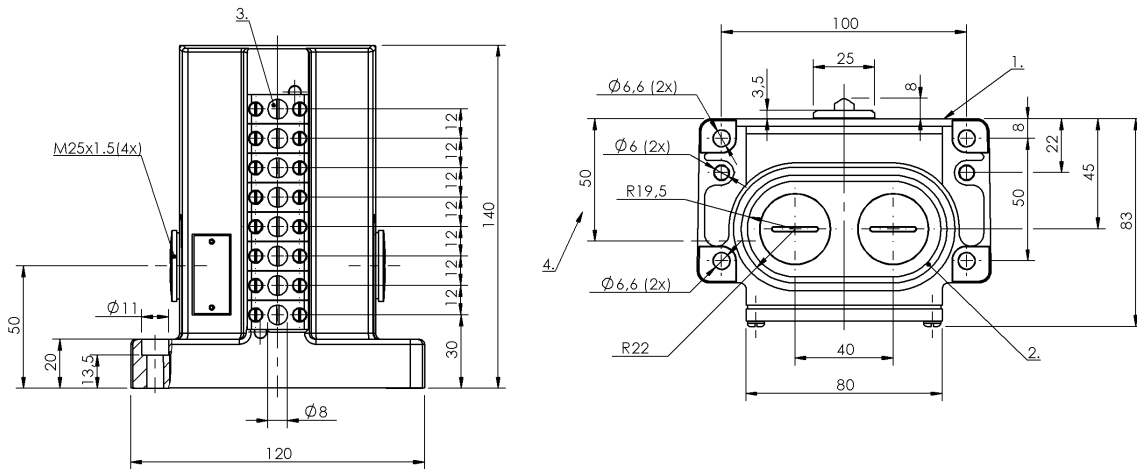
1) Krawędź odniesienia 2) Pierścieni uszczelniający 3) Suwak zapobiegający krystalizacji 4) Przepust kablowy
