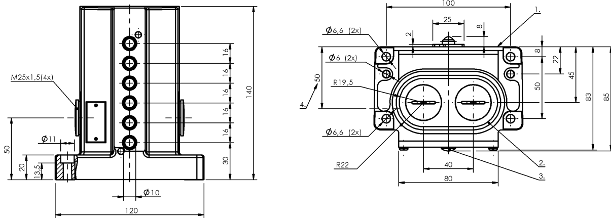
1) Krawędź odniesienia 2) Pierścień uszczelniający 3) Wskazanie funkcji FD/FE/LL 4) Przepust kablowy
