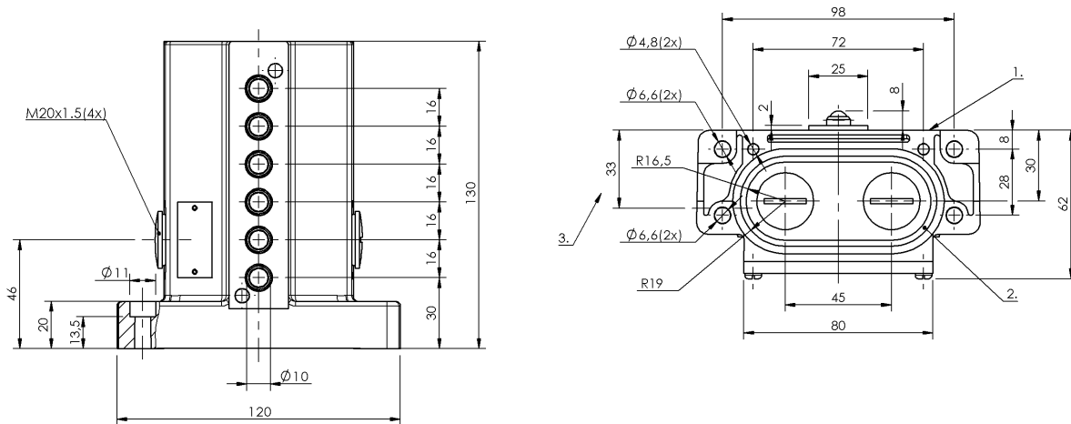
1) Krawędź odniesienia 2) Pierścień uszczelniający 3) Przepust kablowy
