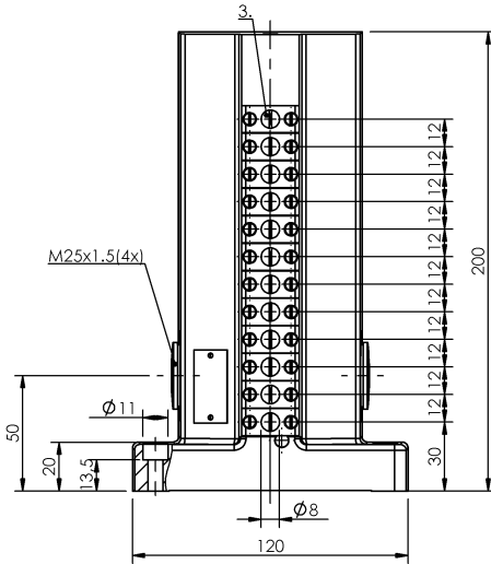
1) Krawędź odniesienia 2) Pierścieni uszczelniający 3) Suwak zapobiegający krystalizacji 4) Przepust kablowy
