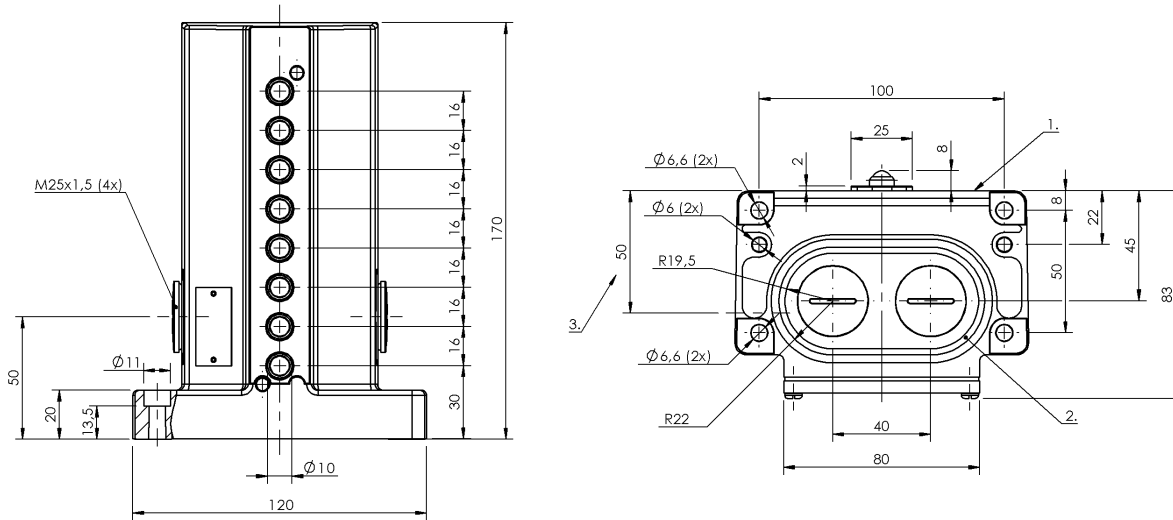
1) Krawędź odniesienia 2) Pierścień uszczelniający 3) Przepust kablowy
