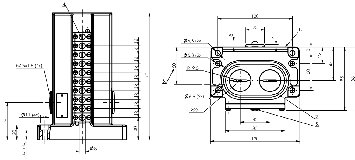
1) Krawędź odniesienia 2) Pierścień uszczelniający 3) Przepust kablowy 4) Suwak zapobiegający krystalizacji 5) Wskazanie funkcji FD/FE/LL
