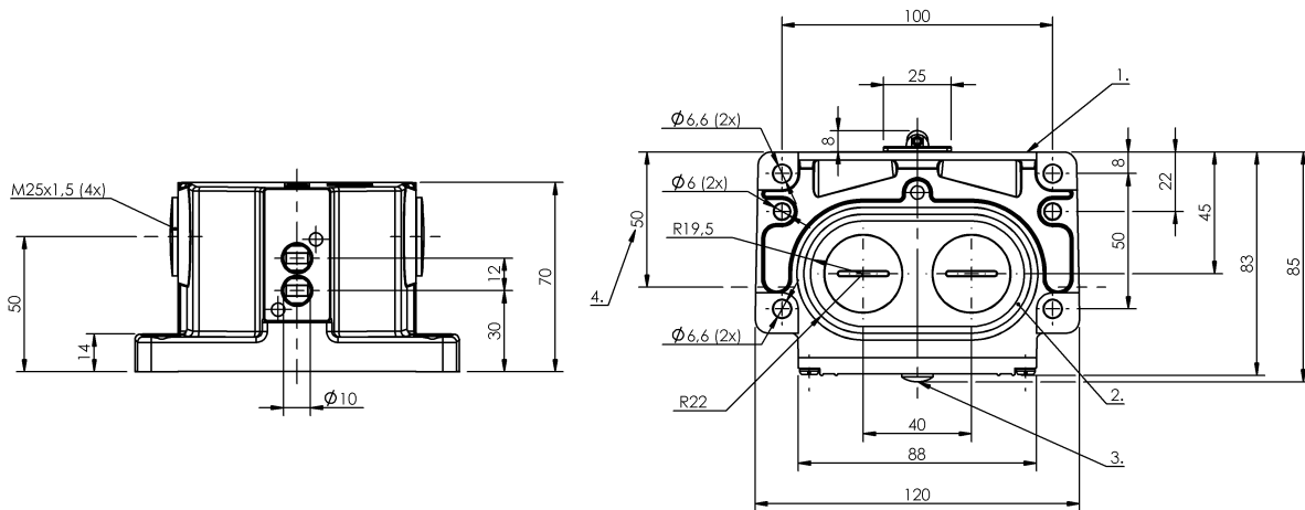
1) Krawędź odniesienia 2) Wskazanie funkcji FD/FE/LL 3) Pierścień uszczelniający 4) Przepust kablowy
