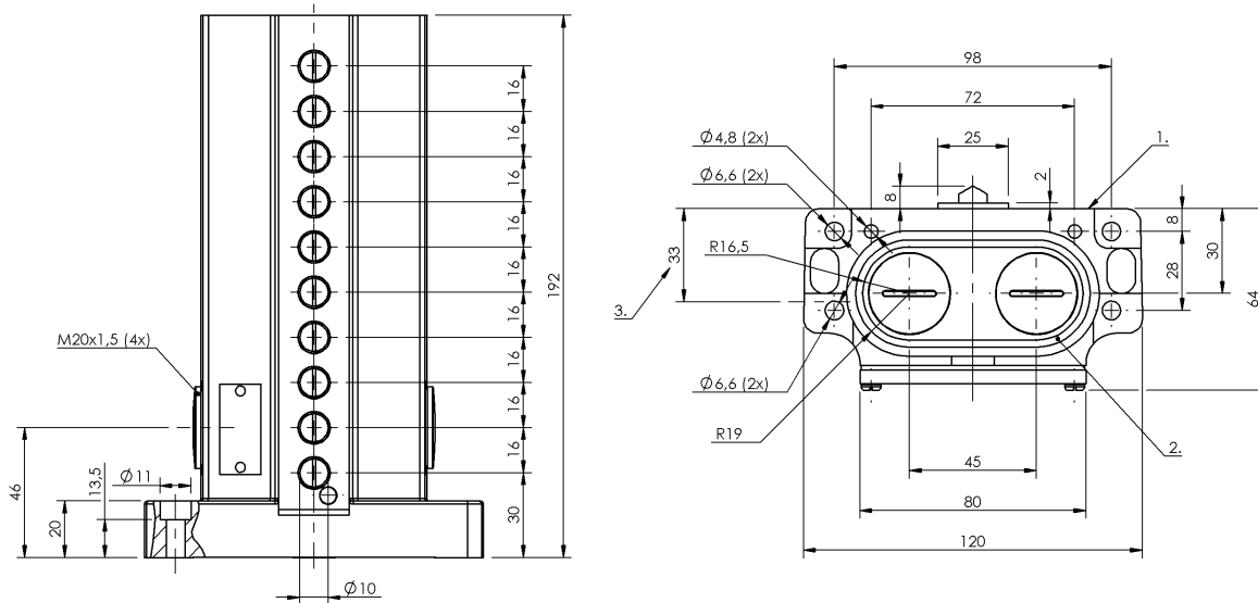
1) Krawędź odniesienia 2) Pierścieni uszczelniający 3) Przepust kablowy
