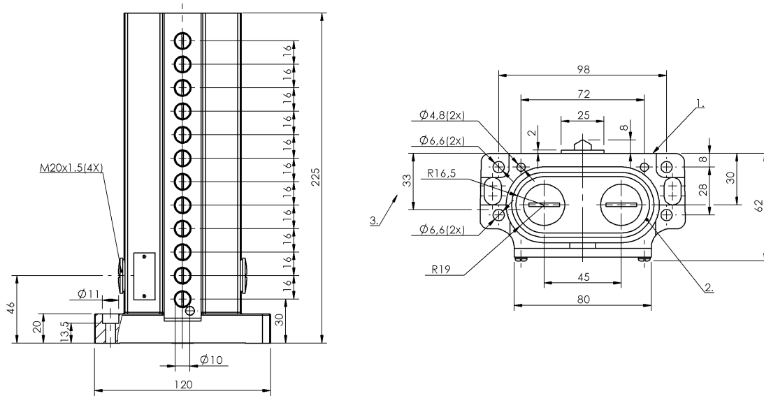
1) Krawędź odniesienia 2) Pierścień uszczelniający 3) Przepust kablowy
