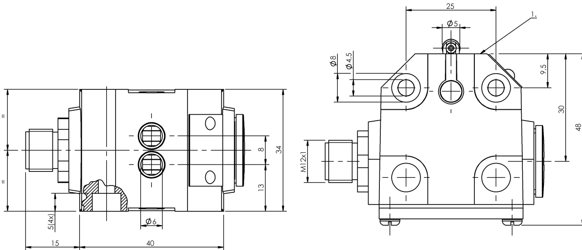
1) Krawędź odniesienia
