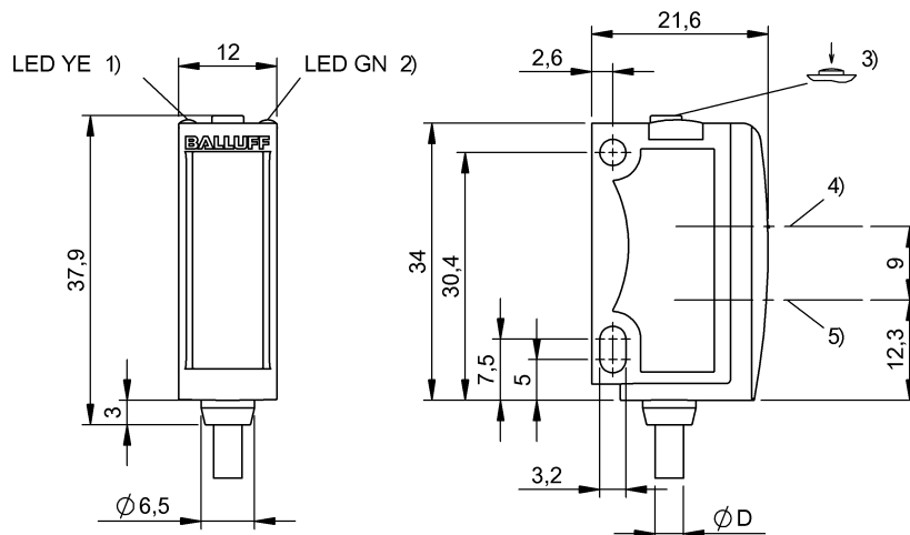
1) Funkcja wyjścia 2) Napięcie robocze 3) Czulość, jasno/ciemno 4) Oś optyczna odbiornika 5) Oś optyczna nadajnika
